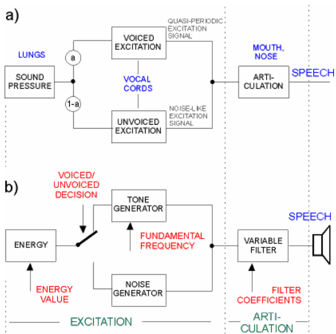
Фиг. 20-24. Машинен модел на устройство на речеви апарат.
