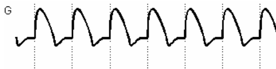
Фиг. 20-22. Импулсна характеристика на звук G.
