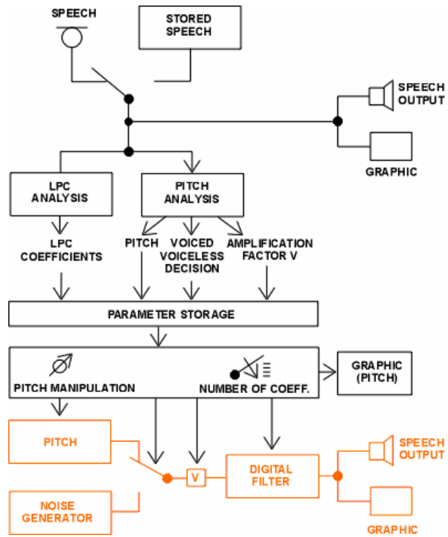
Фиг.20-25. Устройство на Vocoder
