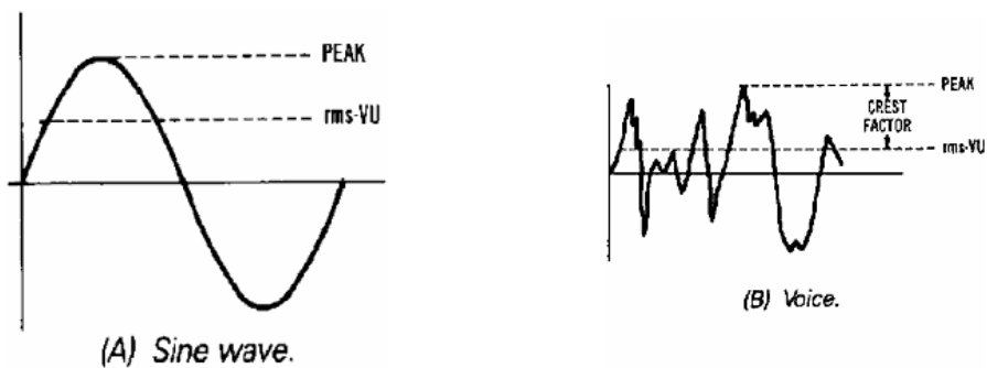
Фиг. 21-2. Крест-фактор на музикален сигнал.
